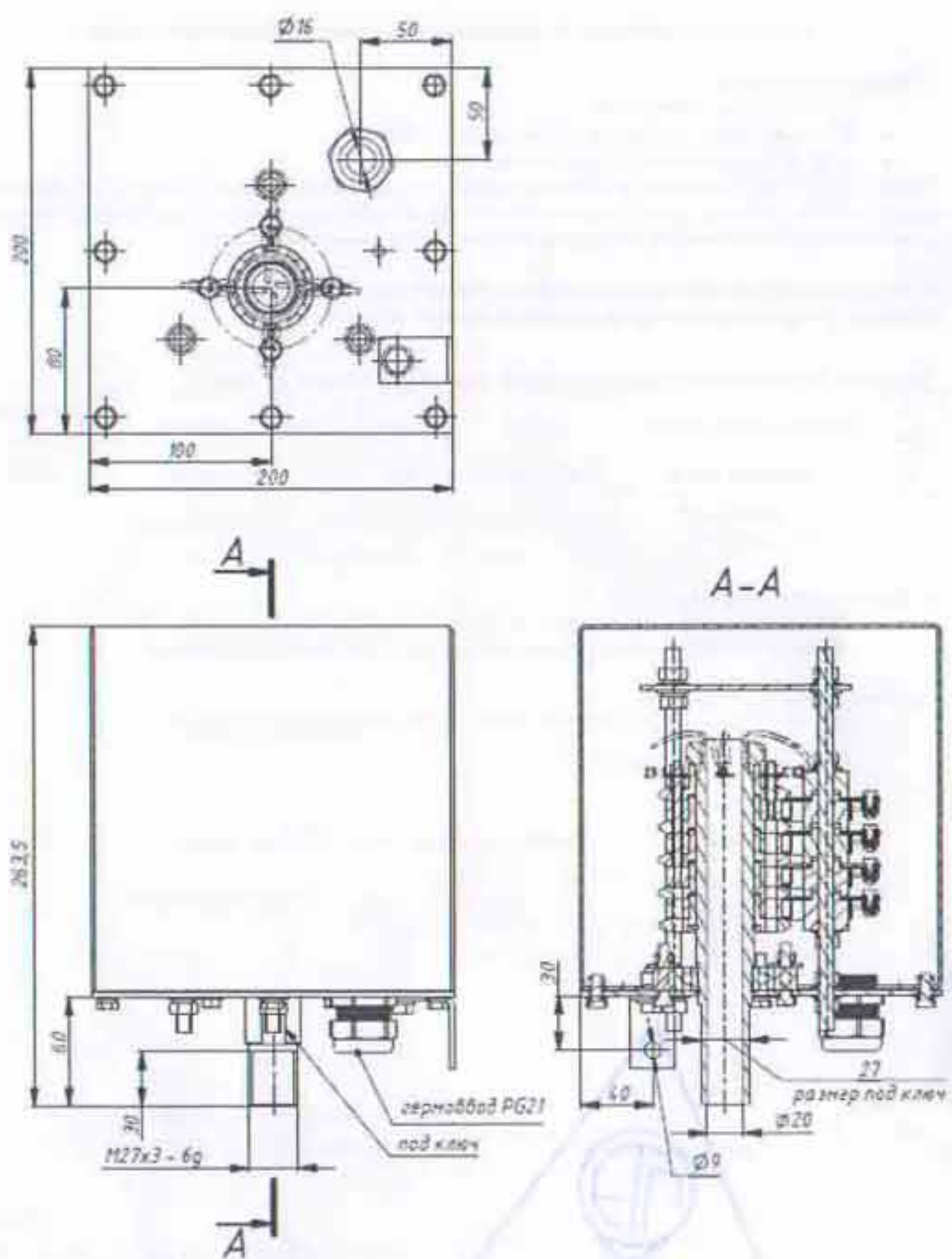
Рис.1 Общий вид и габаритные размеры кольцевого токосъемника
