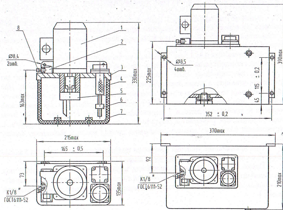
Рисунок 1 – Станция смазочная И-СЭ-2,5/0,5
