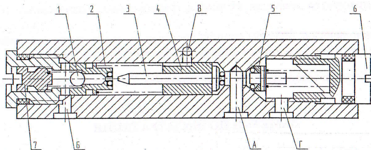
Рисунок 3 – Клапанная коробка
